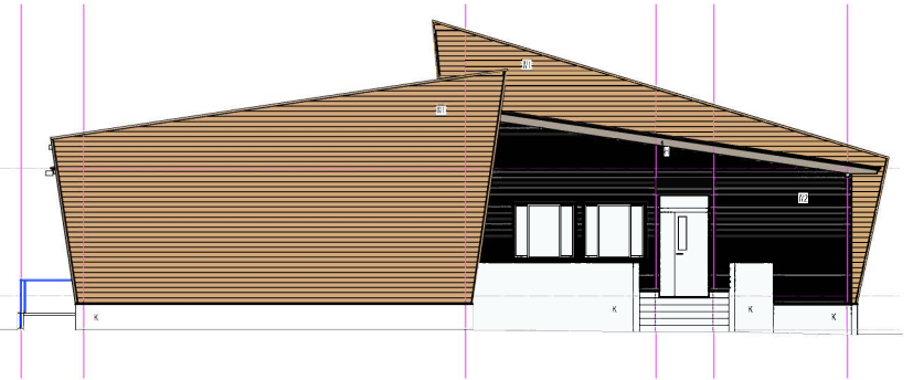
西 立面図
