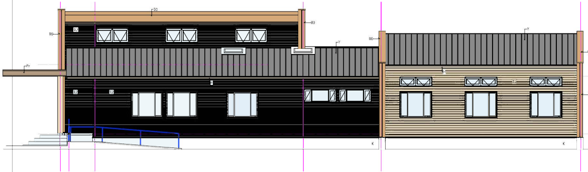
北 立面図
